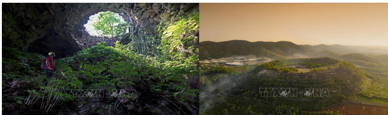
Hình 8. Vùng lõi hang động núi lửa.
